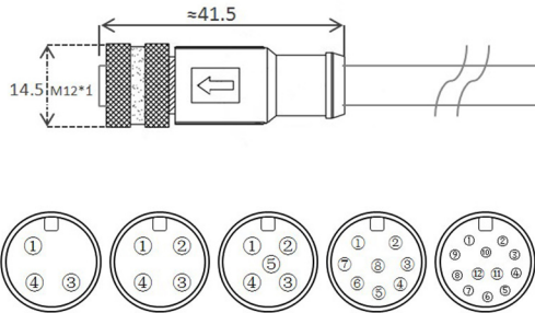
尺寸图
