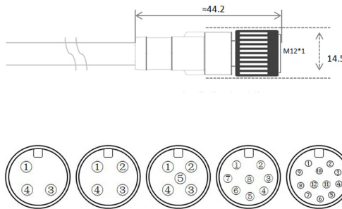
尺寸图 Drawing
