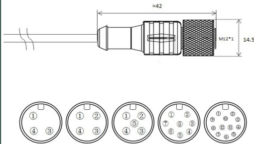
尺寸图
